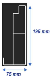
HLINÍKOVÝ PROFIL
